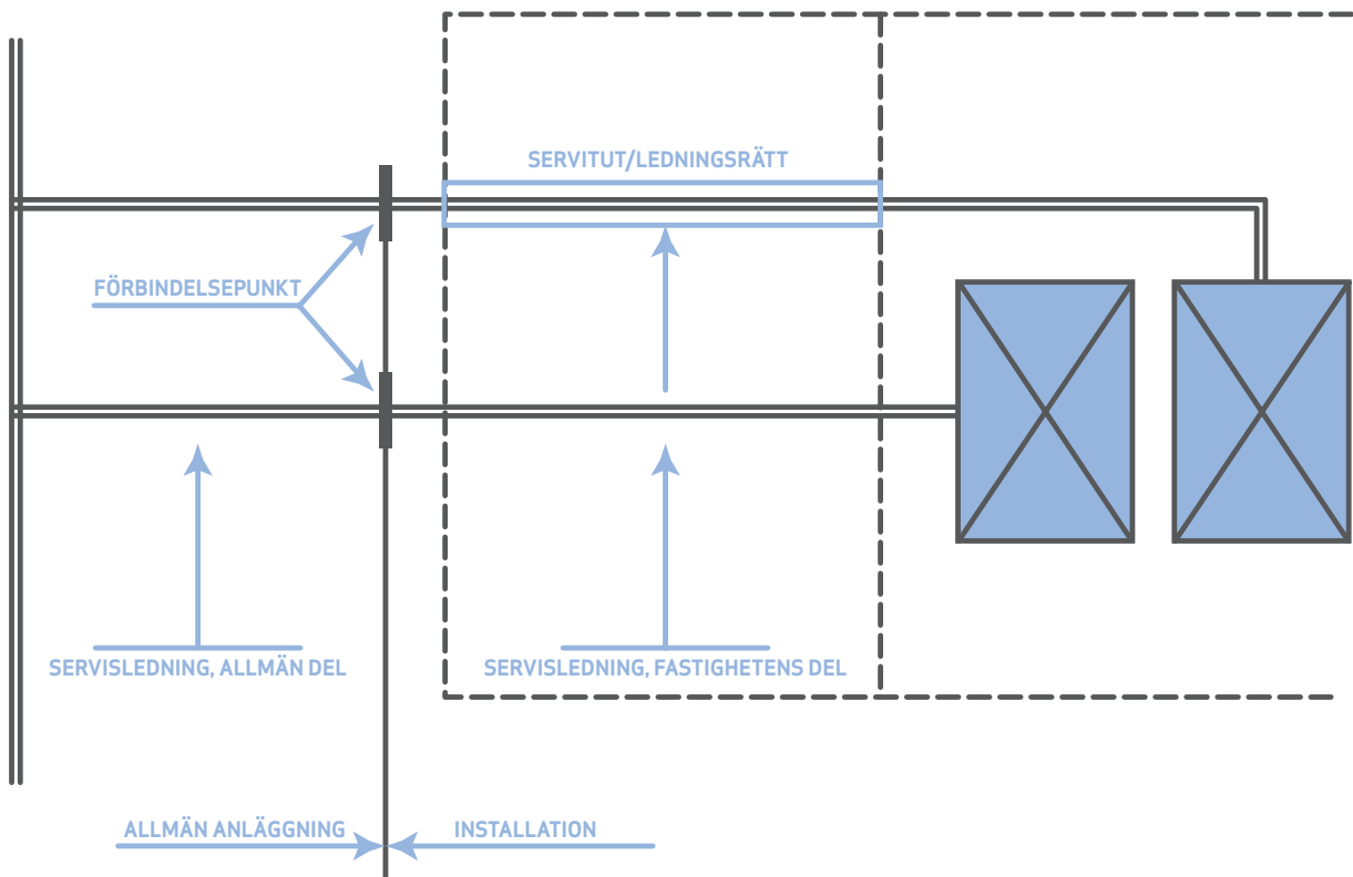
Bild 2 Förbindelsepunkters läge vid fastighet med ledning över annans fastighet
